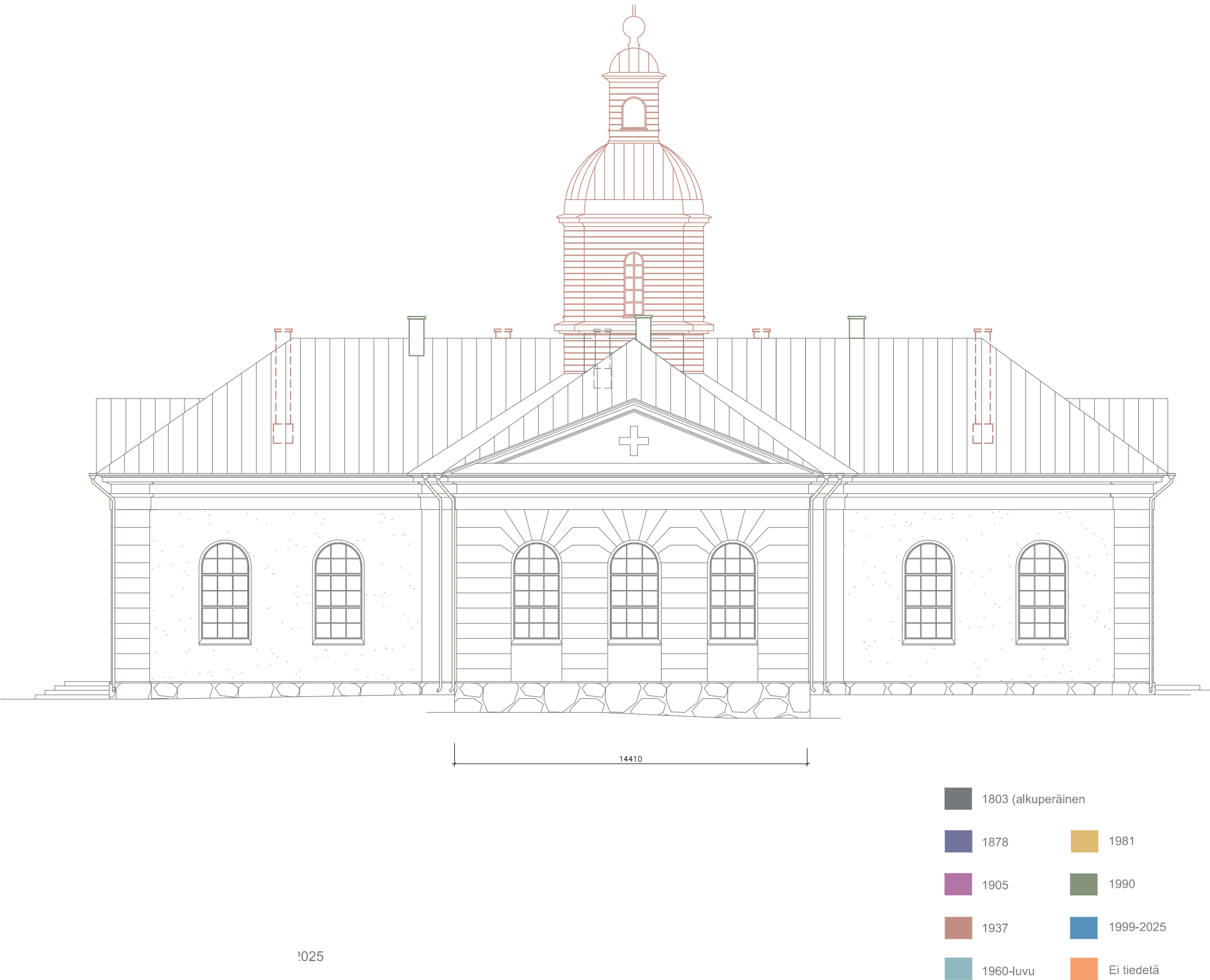
Vähänkyrön kirkko, kronologinen julkisivupiirustus itään (NAC Arkkitehdit, 2025)
