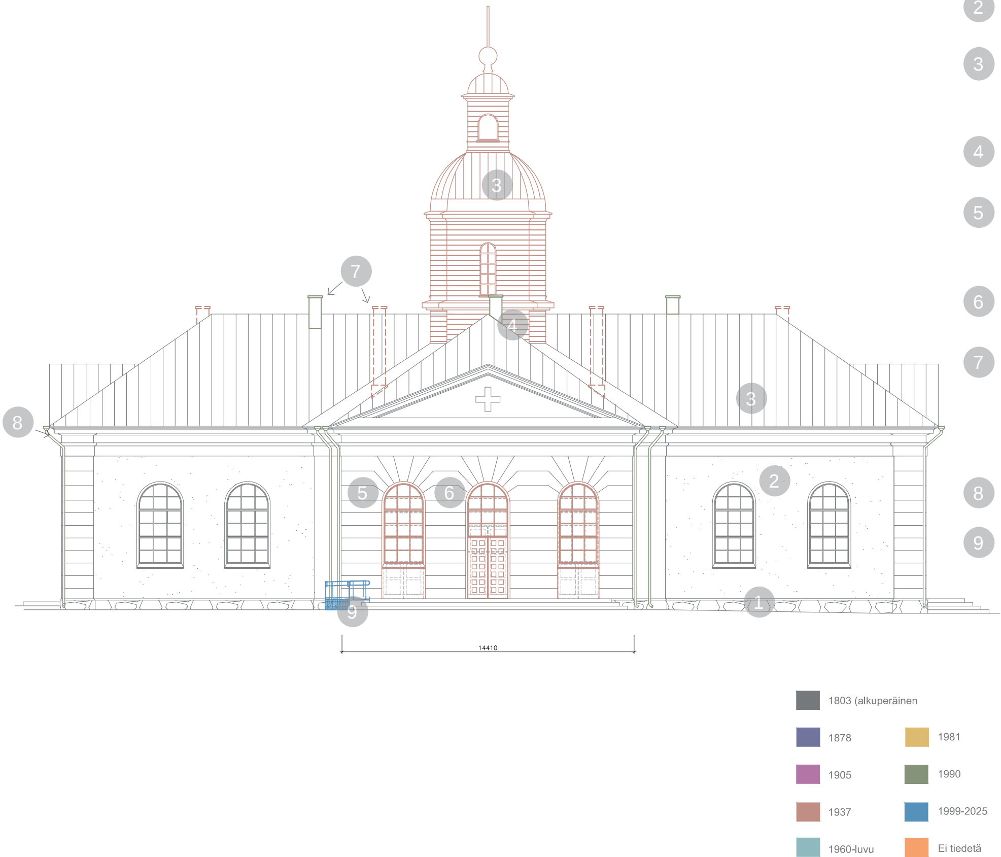
Vähänkyrön kirkko, kronologinen julkisivupiirustus länteen (NAC Arkkitehdit, 2025)
