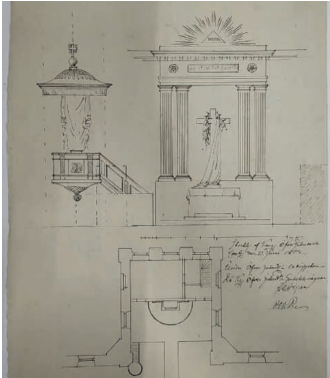
Saarnastuoli ja alttarin piirustus (Riksarkivet Stockholm, tekijä Olof Tempelman, 1786)
