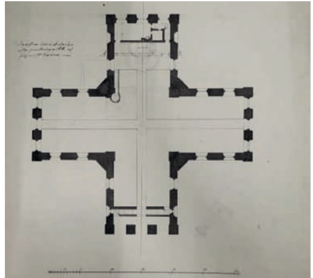
Olof Tempelmanin alkuperäinen pohjapiirustus 1786 (Riksarkivet Stockholm, tekijä Olof Tempelman, 1786)
