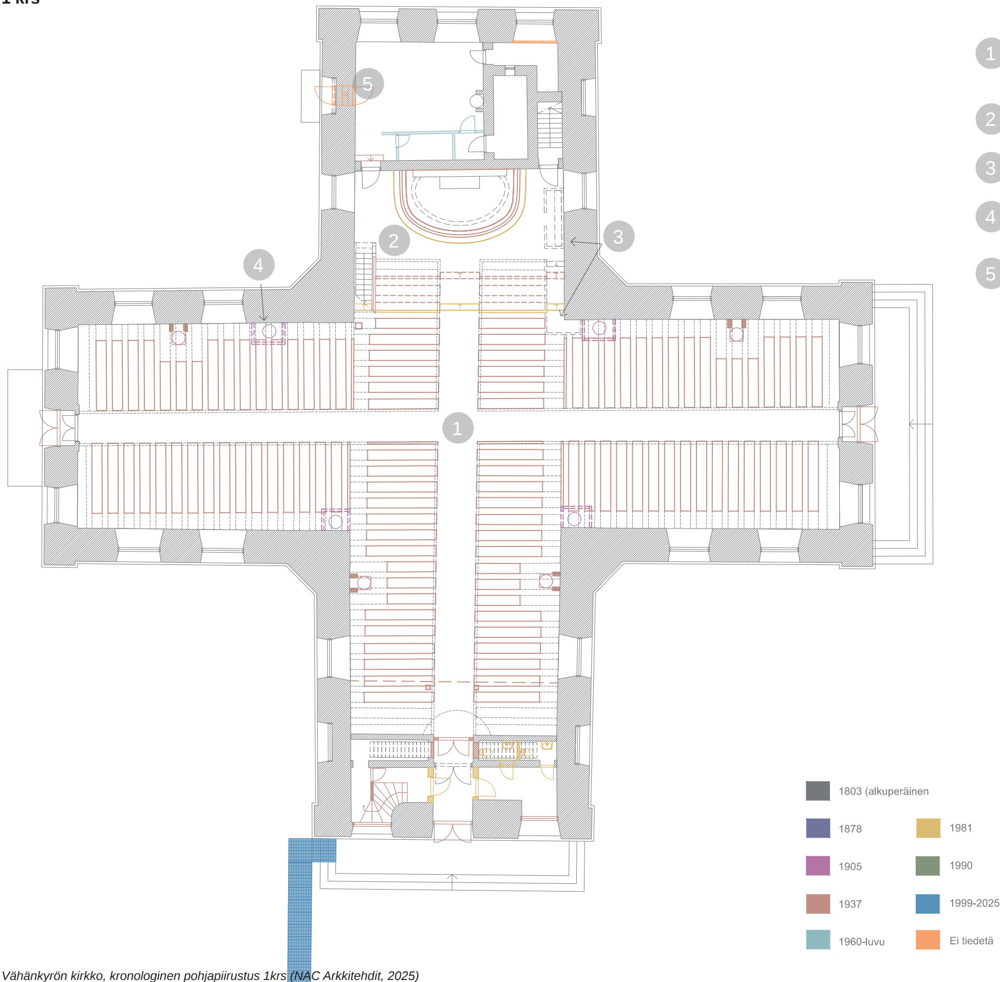
Vähänkyrön kirkko, kronologinen pohjapiirustus 1krs (NAC Arkkitehdit, 2025)
