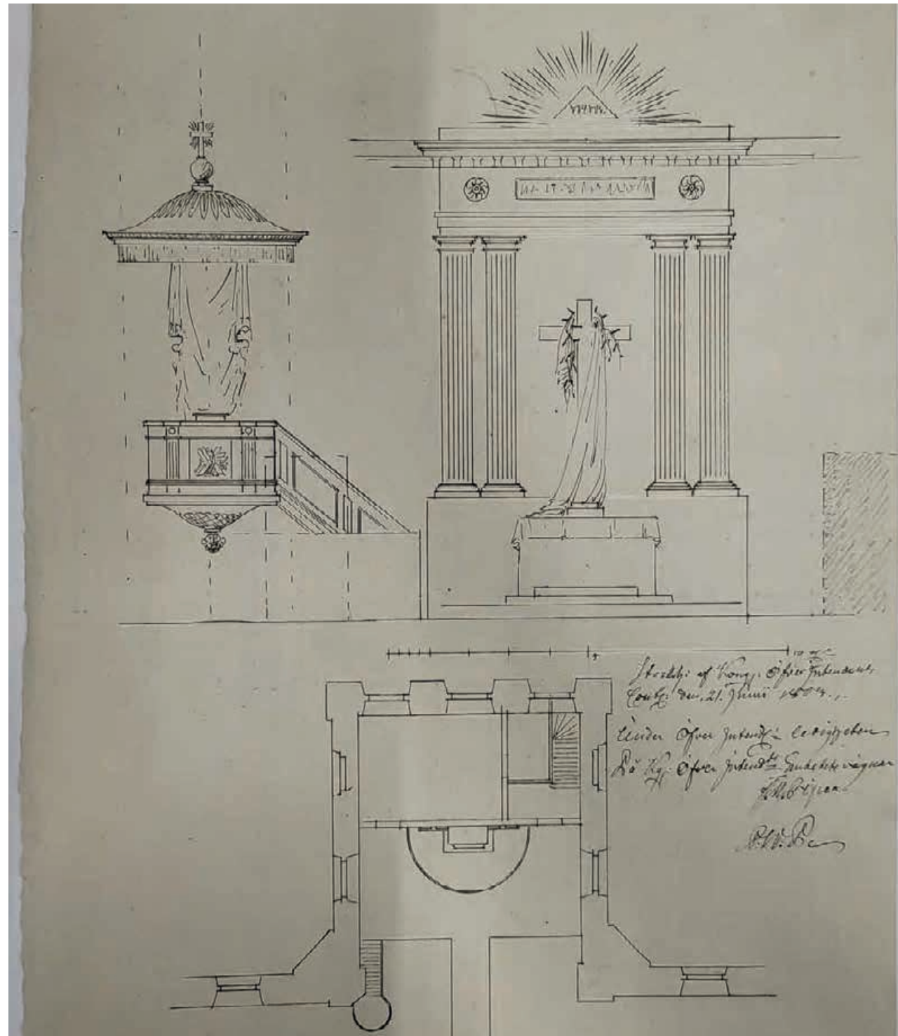
Saarnastuoli ja alttari piirustus 1786, Lähde: Riksarkivet Stockholm
