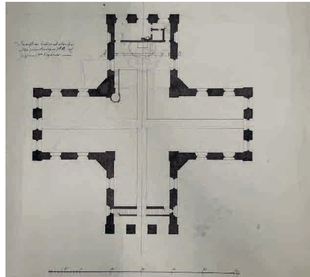
Olof Tempelmanin alkuperäinen pohjapiirustus 1786, Lähde: Riksarkivet Stockholm
